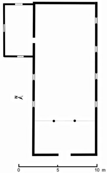
Plan masse de l'édifice
